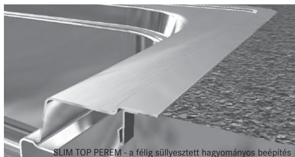
SLIM TOP PEREM - a félig süllyesztett hagyományos beépítés
